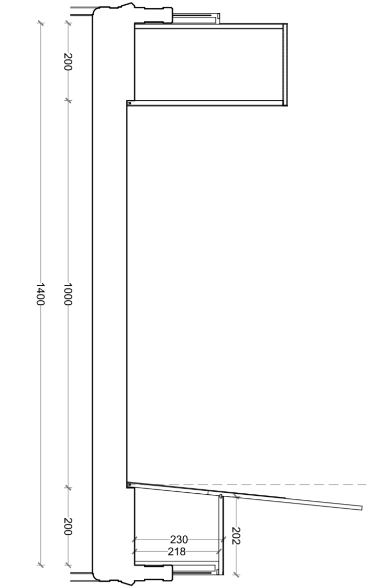
SEZIONE B-B 1:100
