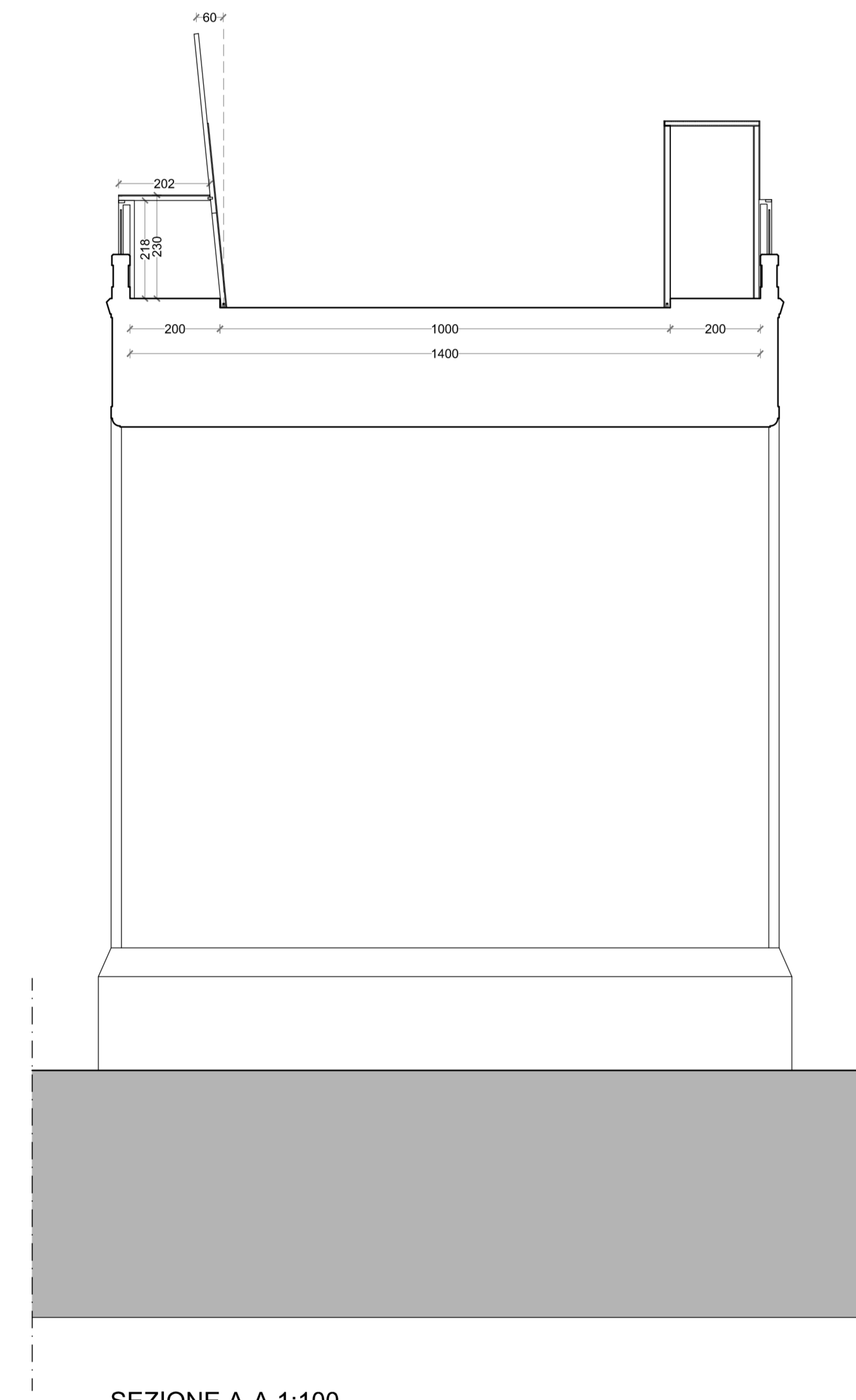
SEZIONE A-A 1:100
