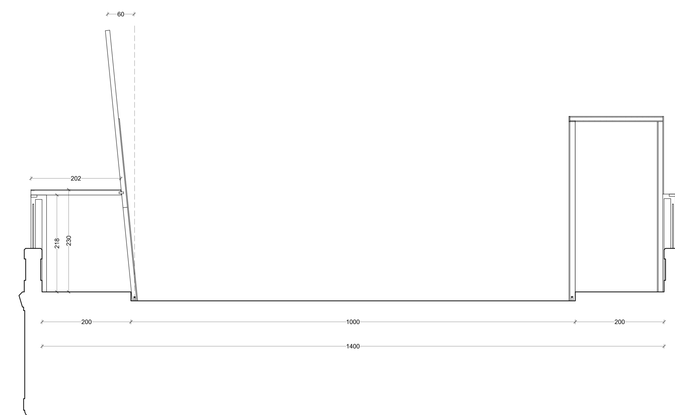
SEZIONE A-A 1:50
